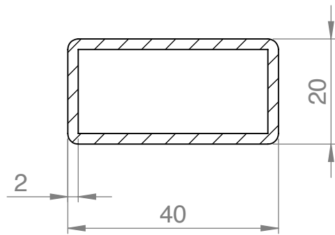
A-A 1:1
